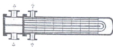
a. U-Tube
