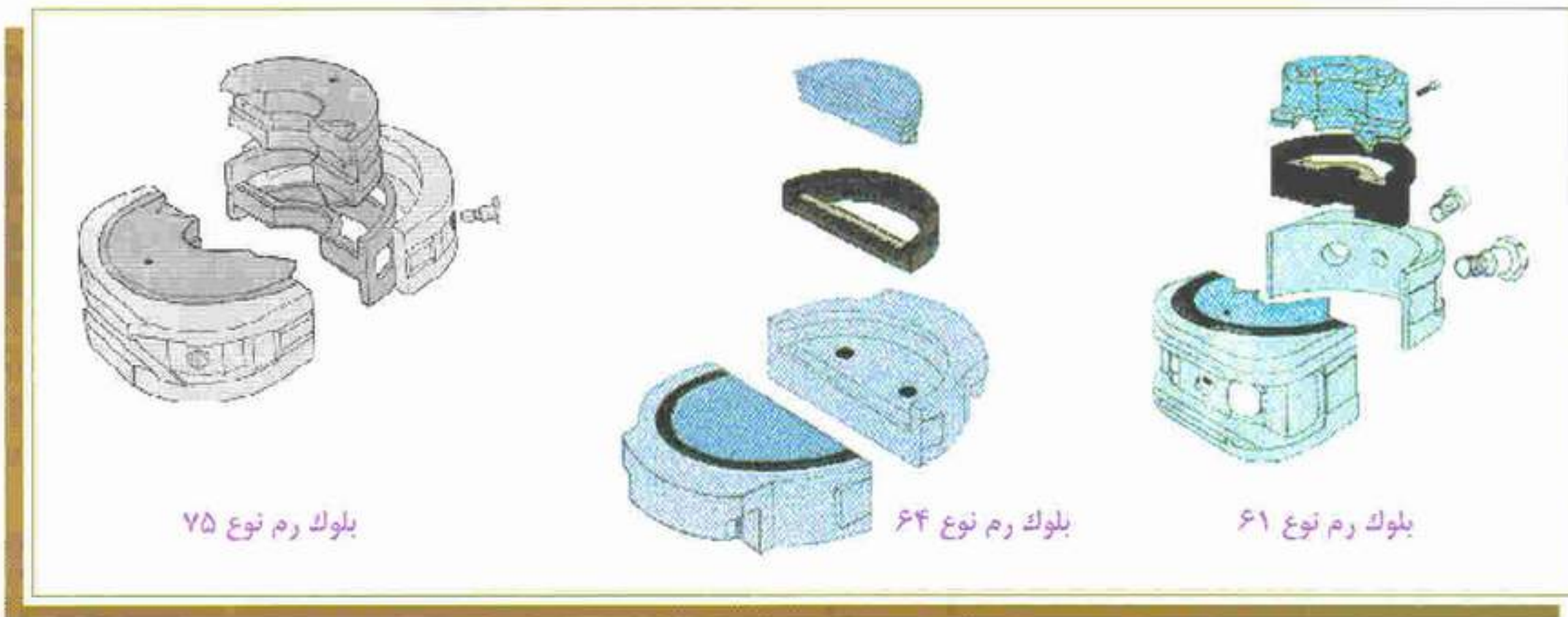
شکل ۱۷- نمایی از چند نوع بلوك رم ساخت شرکت Shaffer
