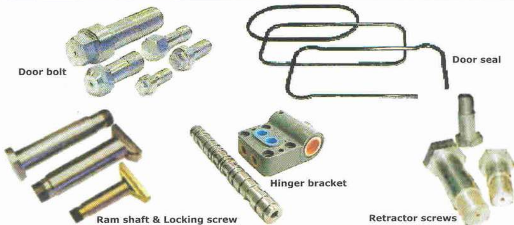
شکل ۱۶- نمای نزدیک از بعضی از قطعات BOP نوع رم
