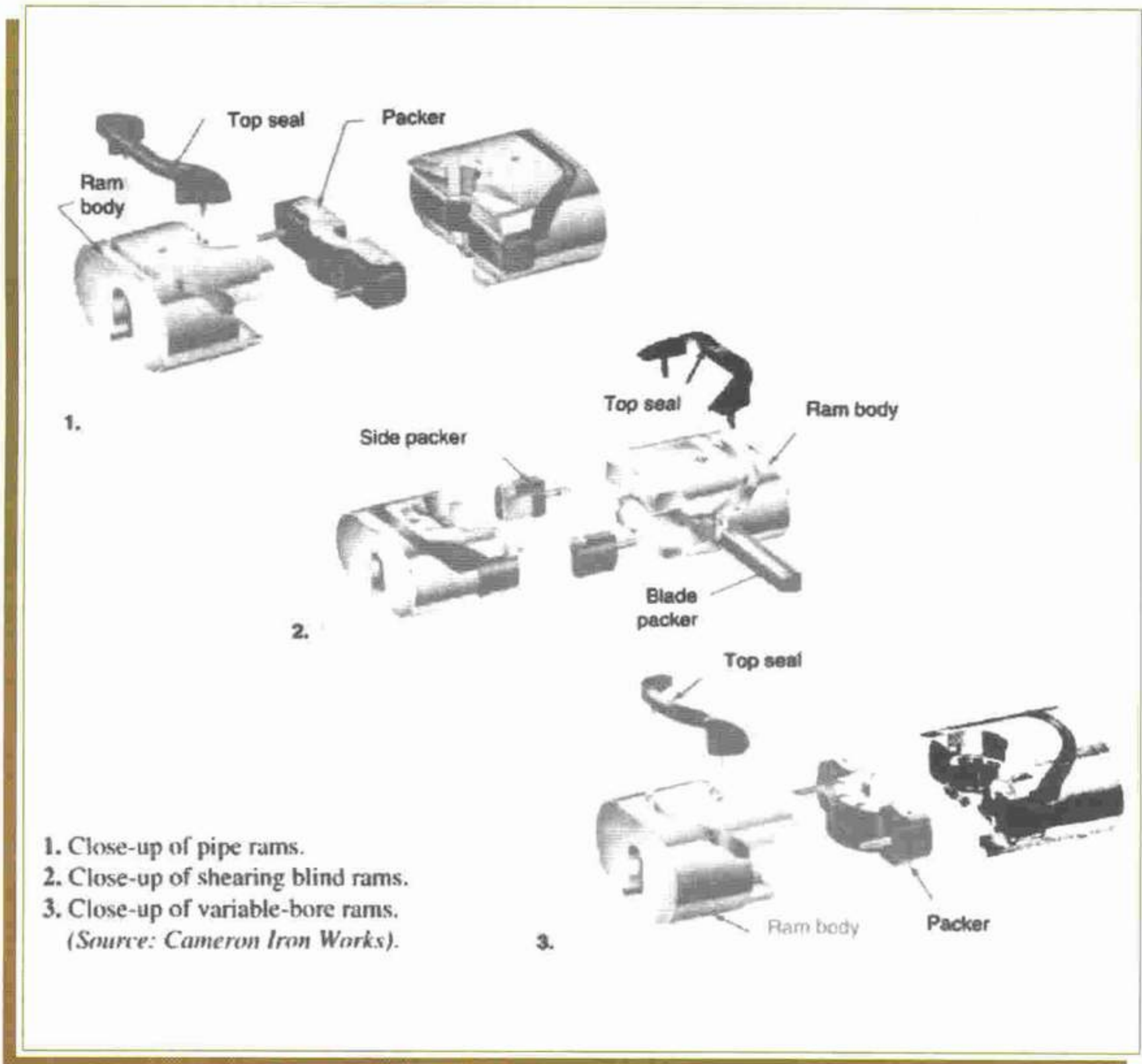
شکل ۱۴- اجزای تشکیل دهنده مجرا بندهای (Packers) رم های نوع لوله ای تخت و تخت برشی
