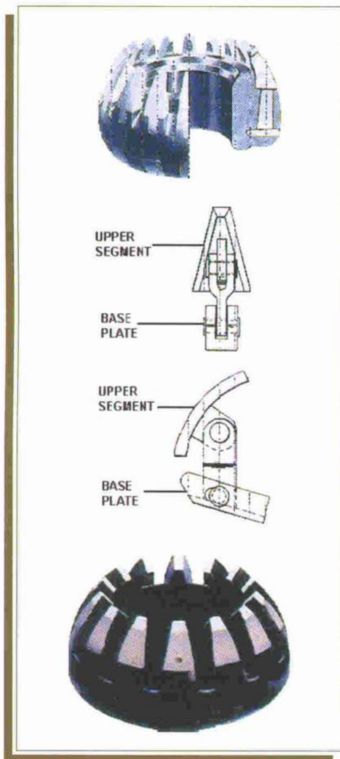
شکل ۶- نمایی از دو نوع المان مسدود کننده
