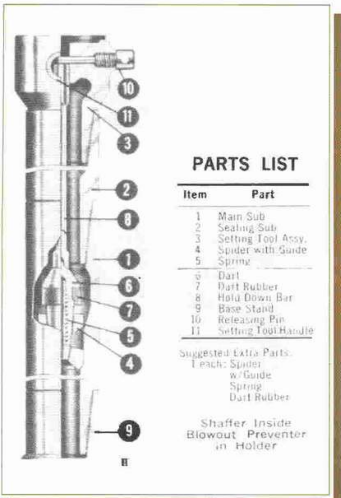
شکل ۲۱- نمایی از یک BOP درونی نوع dart
