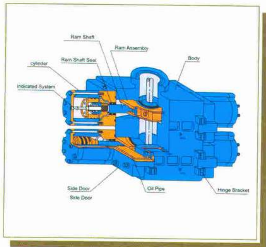
شکل ۱۱- نمایی از یک رم لوله‌ای
