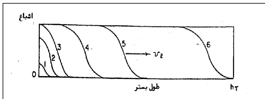
شکل ۵-۶ الف- حرکت ناحیه جذب در طول بستر
