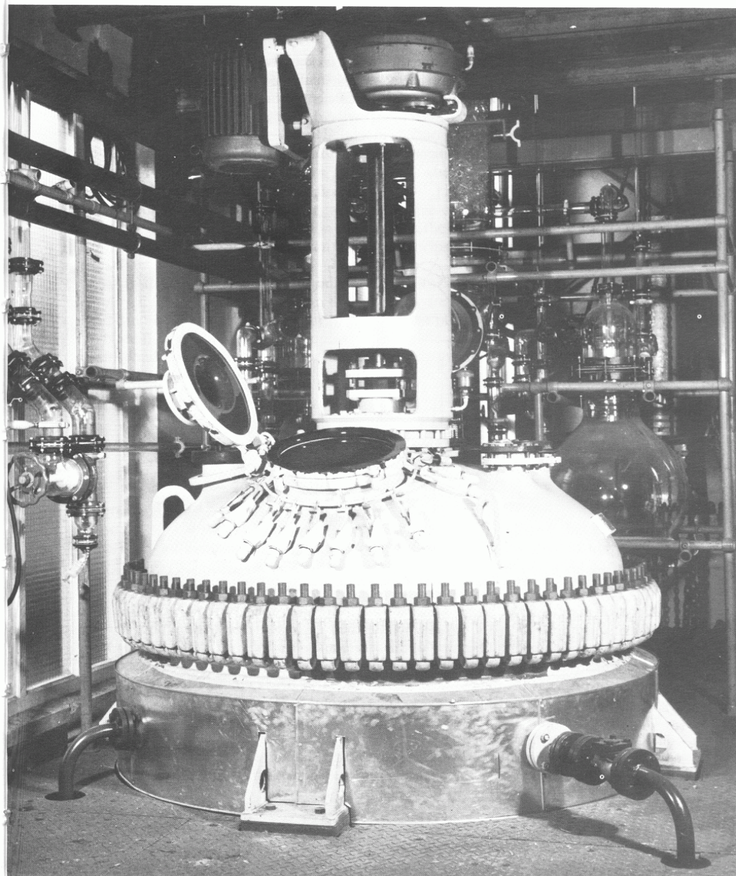
شکل 1-11- تصویری از قسمت فوقانی یک راکتور مخلوط شونده
