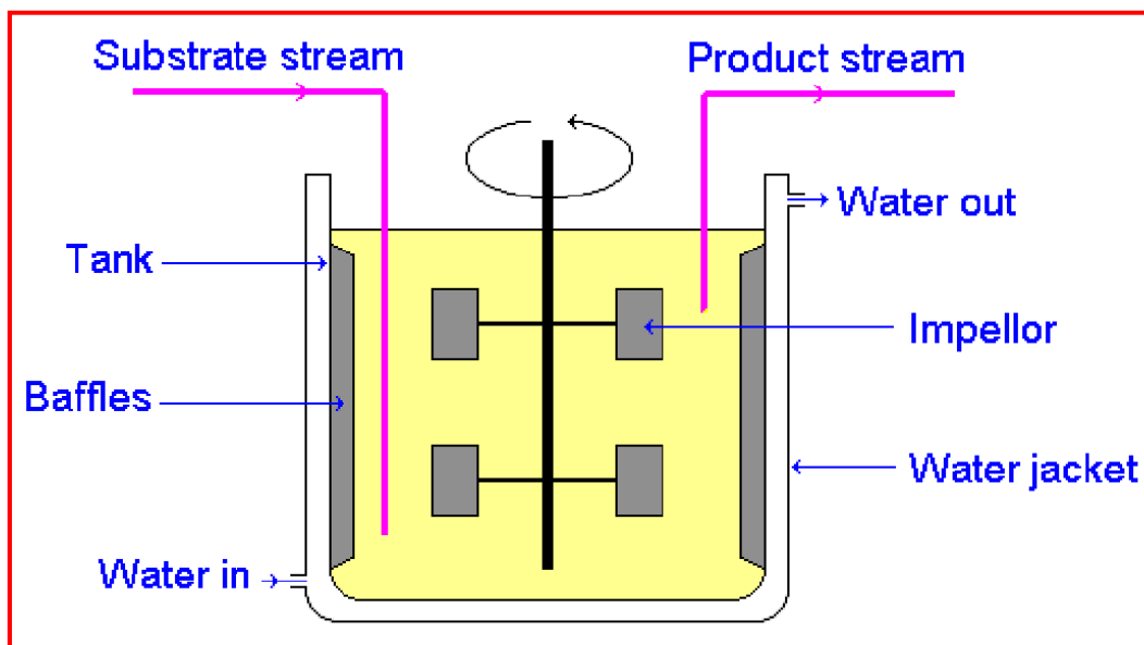
شکل 1-7- راکتور مخلوط شونده
