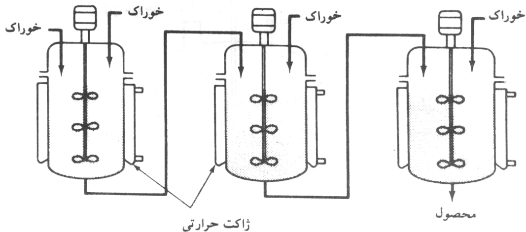
شکل 1-9- سری راکتور مخلوط شونده
