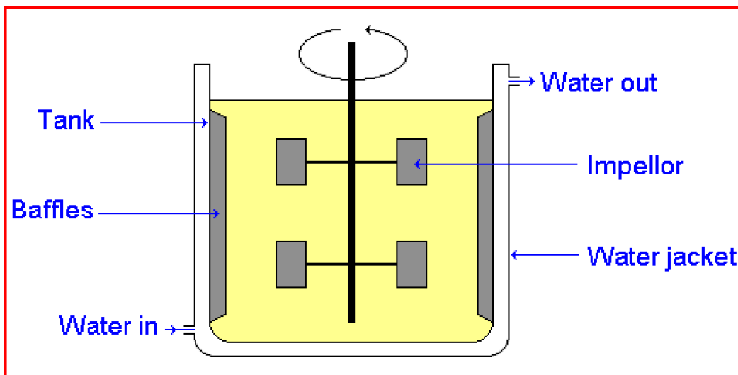
شکل 2-1- راکتور ناپیوسته
