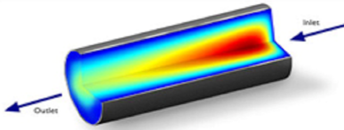
شکل 1-14- نمایش نقاط داغ در یک راکتور لوله‌ای
