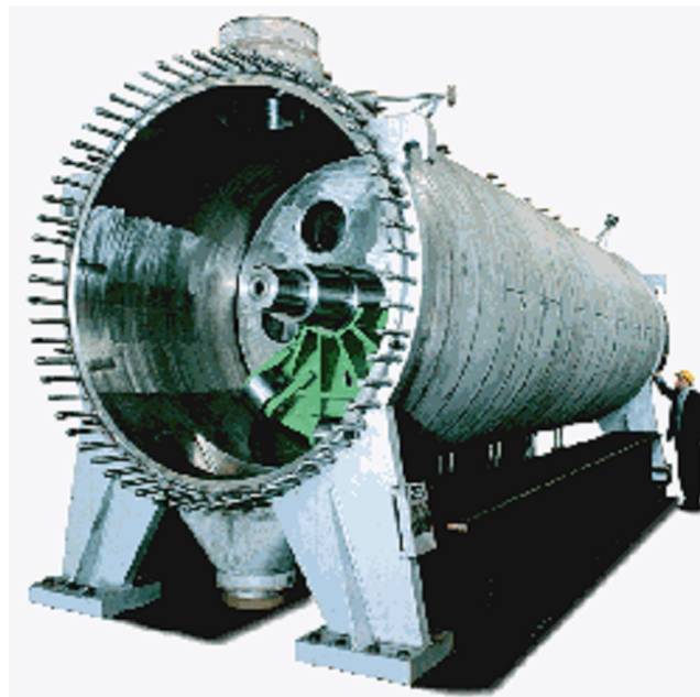
شکل 1-18- شمایی از راکتور لوله ای
