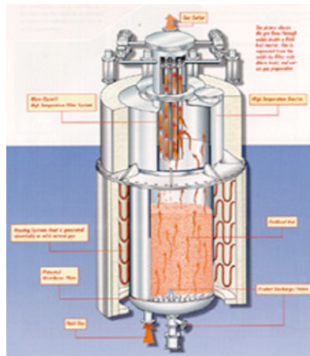
شکل 1-17- راکتور بستر سیال Fluidized Bed Reactor
