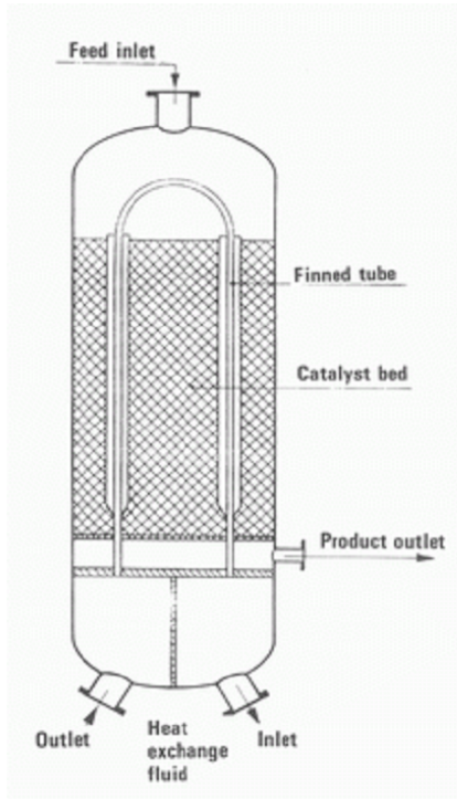
شکل 1-16- راکتور بستر ثابت Fixed Bed Reactor
