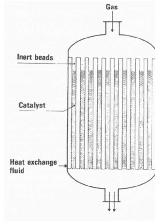
شکل 1-15- راکتور بستر ثابت Fixed Bed Reactor
