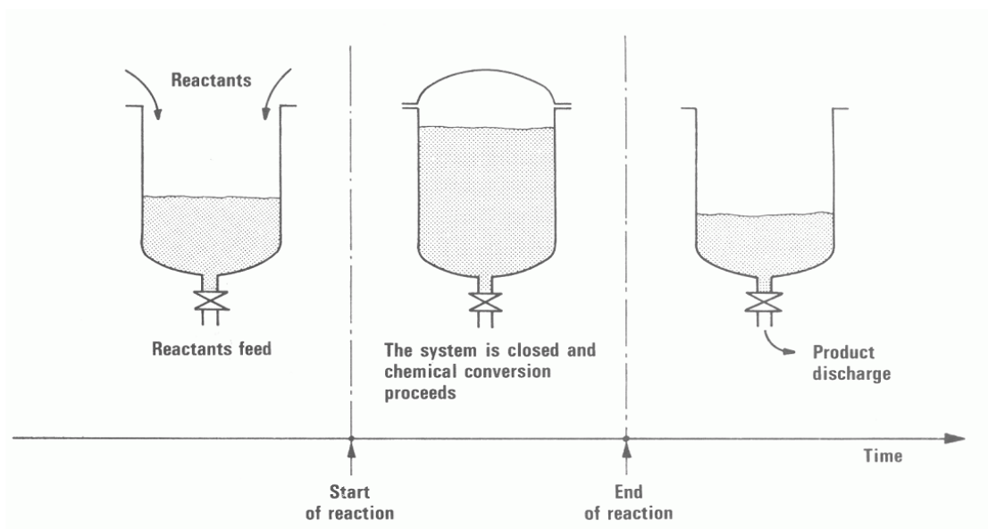
شکل 1-4- مراحل کارکرد یک راکتور ناپیوسته
