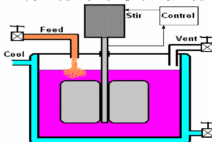
شکل 1-19- راکتور CSTR
